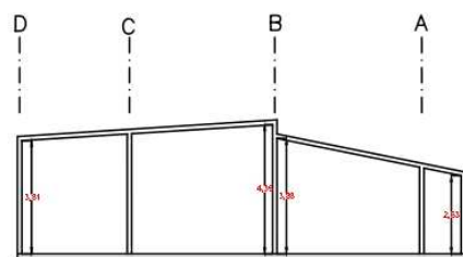
CORTE ESTRUCTURAL
